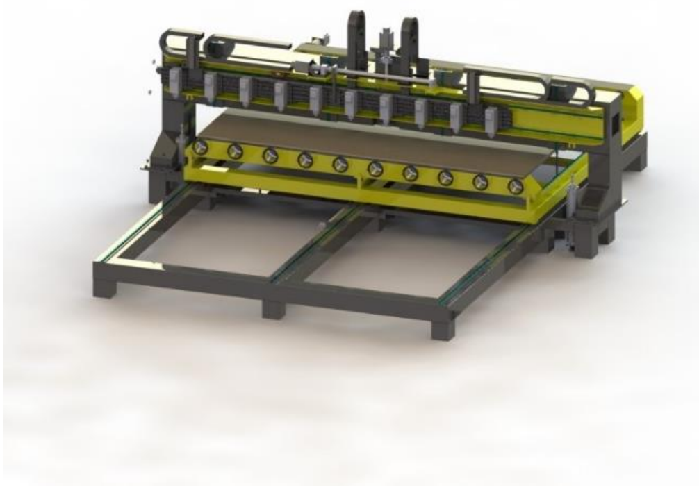
شکل ۱- نمای کلی دستگاه (متحرک بودن محور y )
